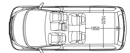
Dubbele Cabine
